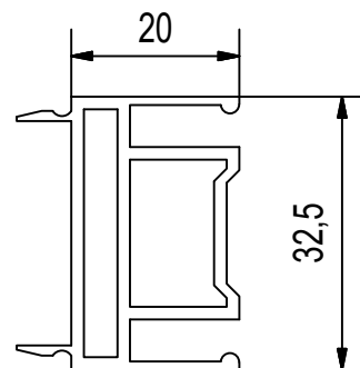
Distanční profil - STF
