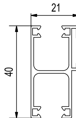
Vodící profil - standardní dvojitý (drážka na střed) typ SDV 2
