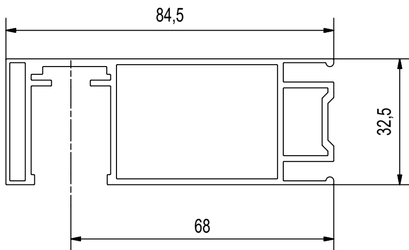
Vodící profil - STF 2
