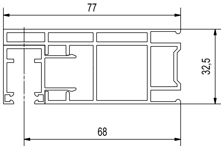
Vodící profil - STF 1
