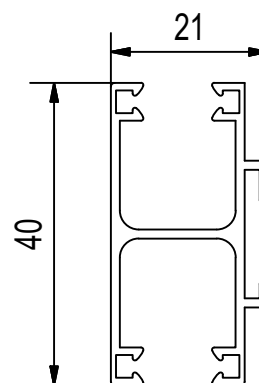
Vodící profil - kulatý dvojitý typ KDV
